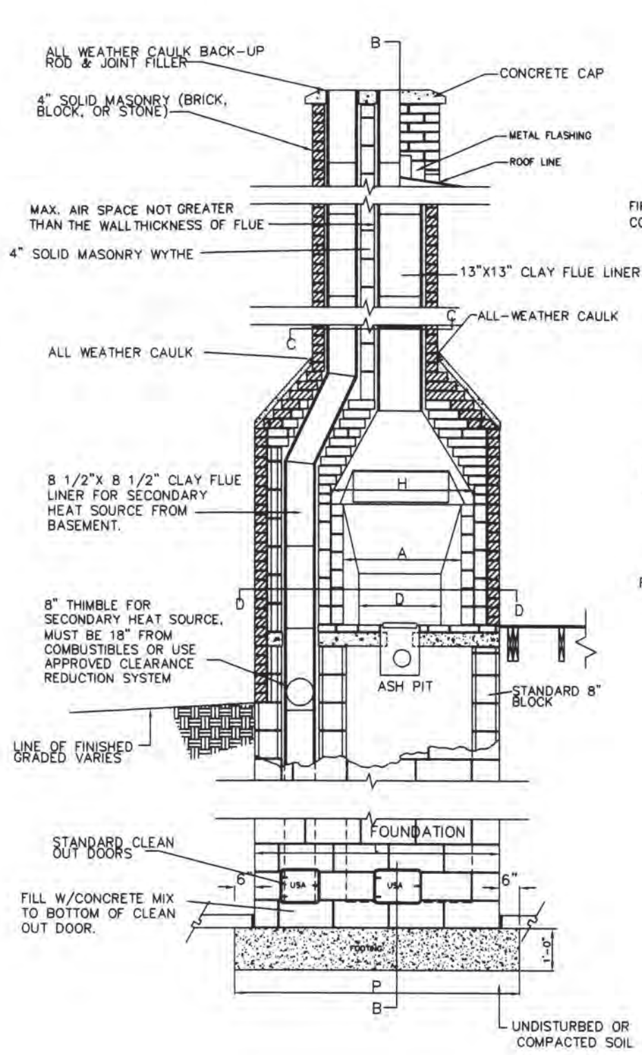
SECTION A-A
